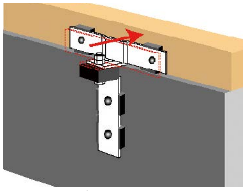
芯々施工の場合はホルダーをスライド(約20mm)させて使用します。
